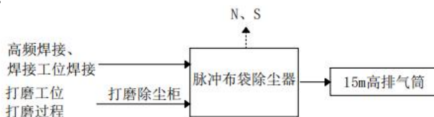
图 9 现有工程焊接、打磨废气处理工艺流程及产排污节点图
