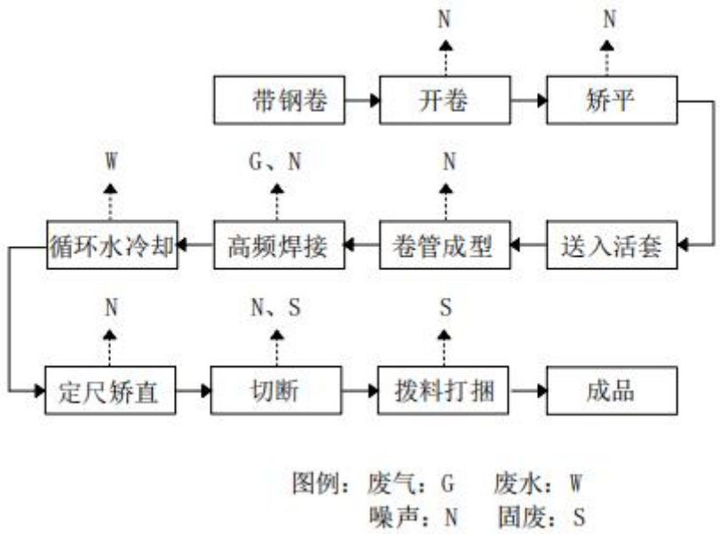
图 3 现有工程钢管加工工艺流程及产排污节点图
