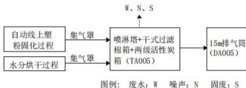
图 37 自动线上塑粉固化过程废气处理工艺流程及产排污节点图
