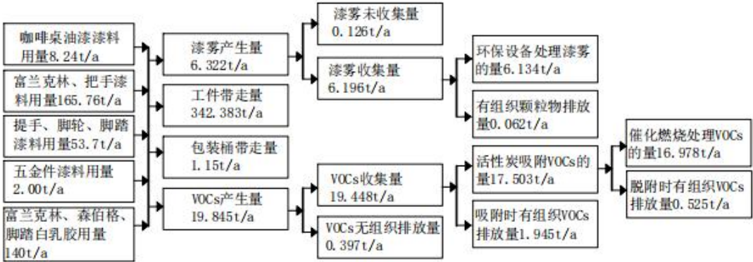
图 12 咖啡桌、富兰克林、脚踏、提手、把手、脚轮、五金件、森伯格 漆料和白乳胶物料平衡图
