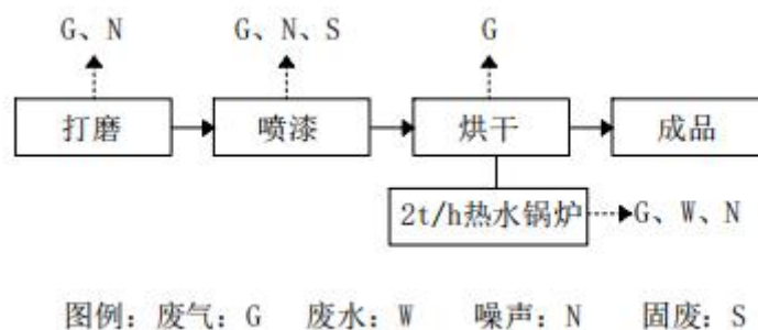
图 2 现有工程木面加工工艺流程及产排污节点图
