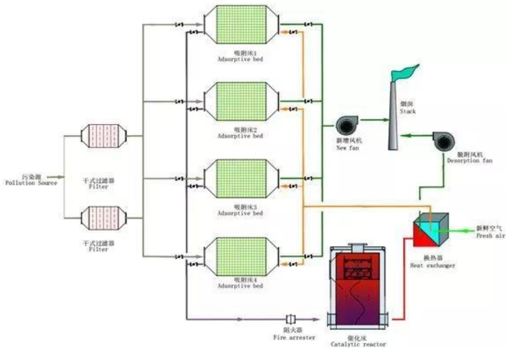
图 54 项目有机废气处理工艺流程图
