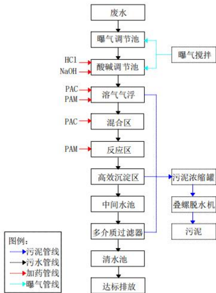
图 55 项目污水处理站工艺流程图
