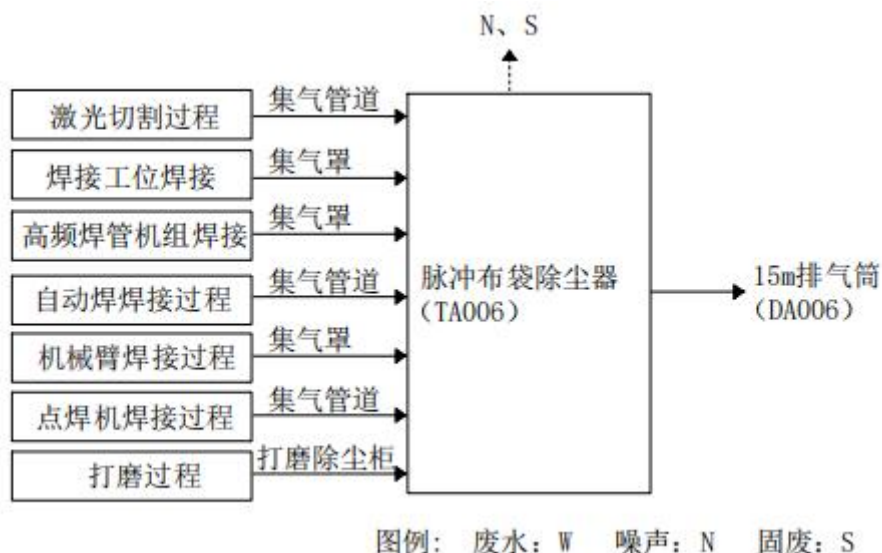
图 38 冲压车间激光切割、焊接、打磨过程废气处理工艺流程及产排污节点图
