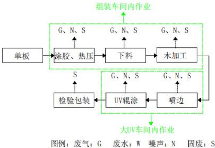
图 22 本项目森伯格椅子面加工工艺流程及产排污节点图
