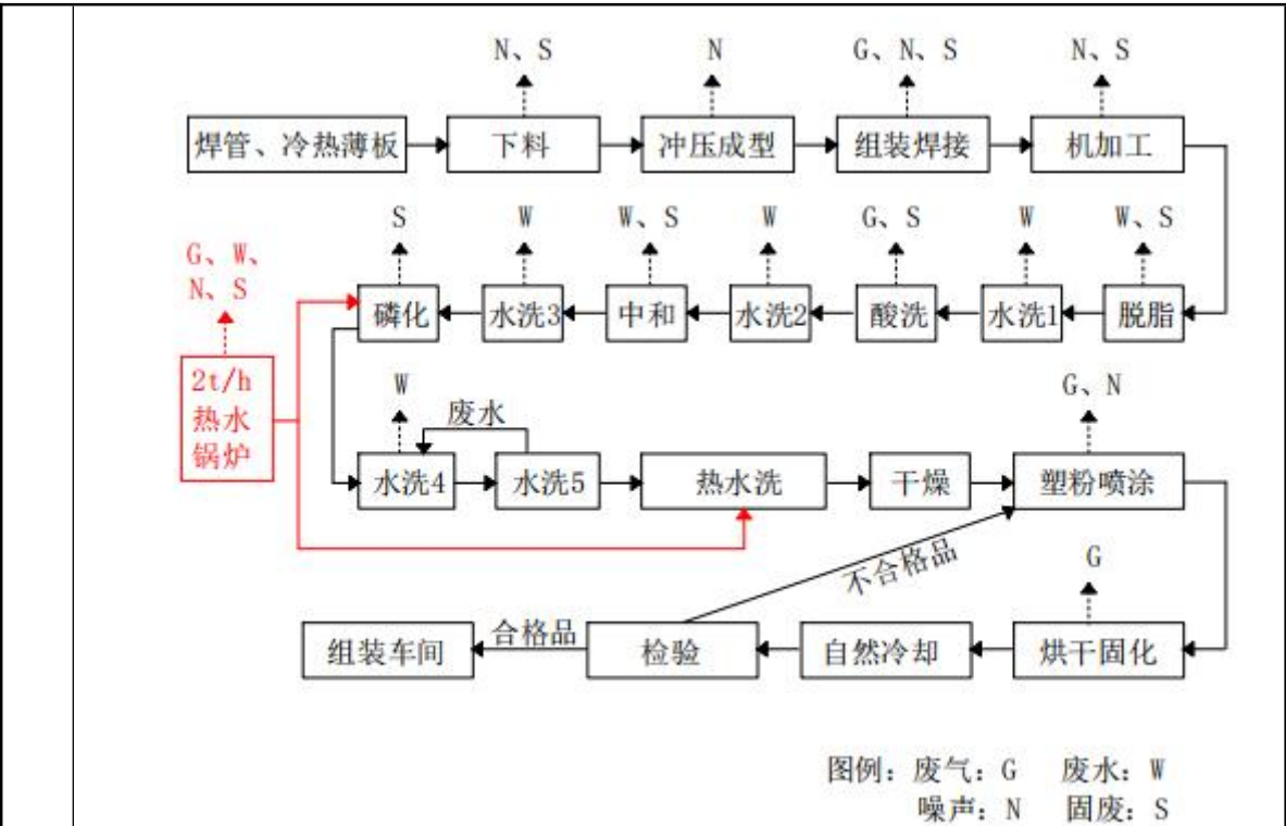
图 4 现有工程钢支架加工工艺流程及产排污节点图
