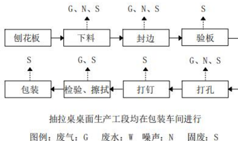
图 20 本项目抽拉桌桌面加工工艺流程及产排污节点图
