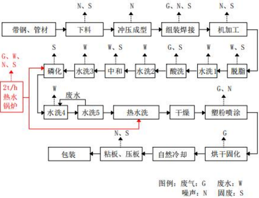
图 5 现有工程篮球架生产工艺流程及产排污节点图
