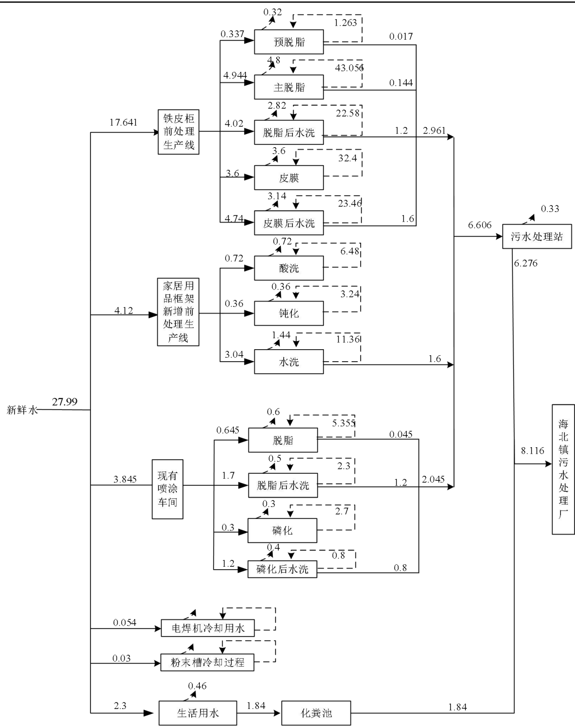
图2-2 项目建成后全厂给排水水量平衡图 单位：m³/d
