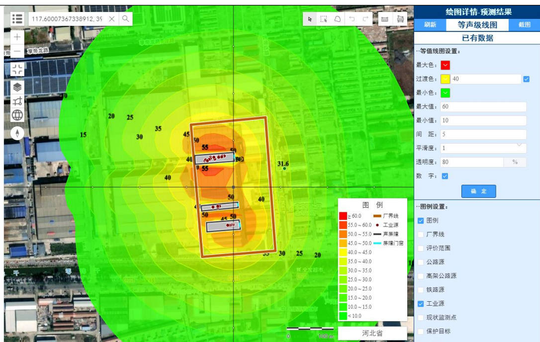
图 4-3 本项目噪声贡献值预测图
