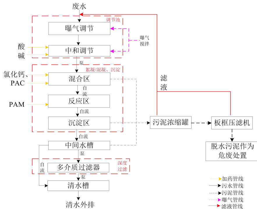
图 4-1 项目污水处理站工艺流程图
