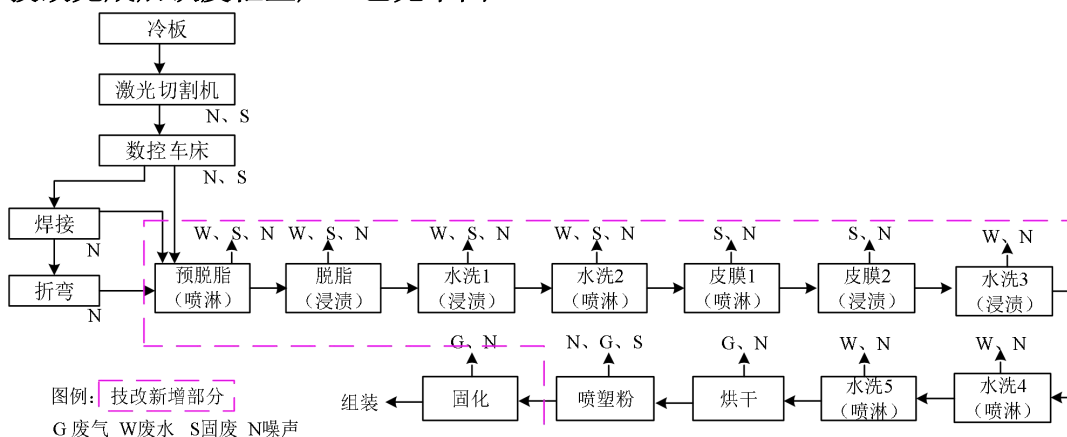
图 2-5 技改完成后铁皮柜生产工艺流程图
