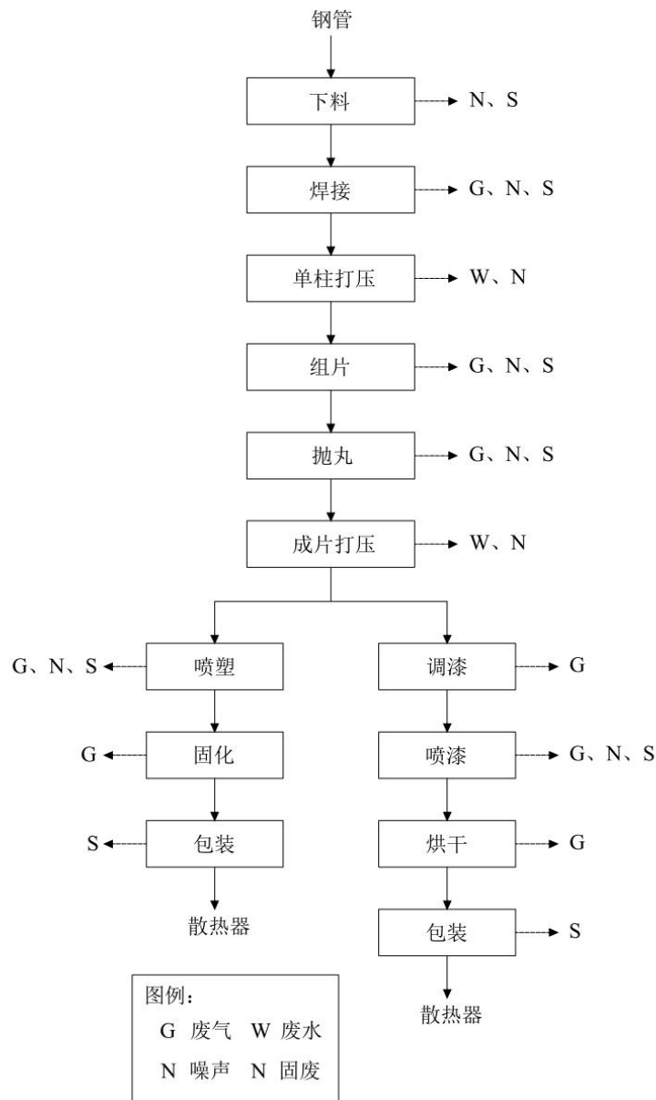
图3 散热器生产工艺流程及排污节点图
