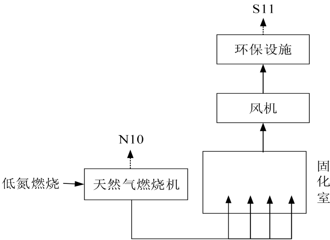
图 2-5 喷涂生产线固化废气走向设施示意图
